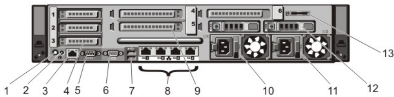
Ilustración 3. Características e indicadores del panel posterior
