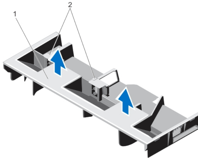
Ilustración 9. Extracción e instalación de la cubierta de refrigeración
