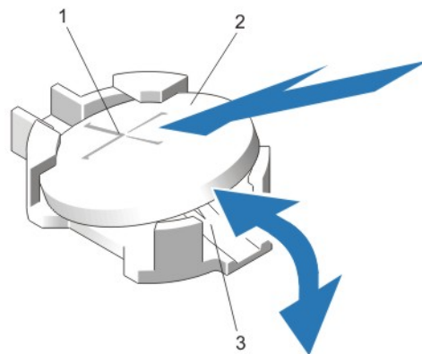
Ilustración 39. Sustitución de la pila del sistema
